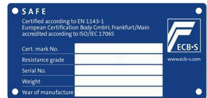
Beispiel Typenschild ECB-S-Tresore
